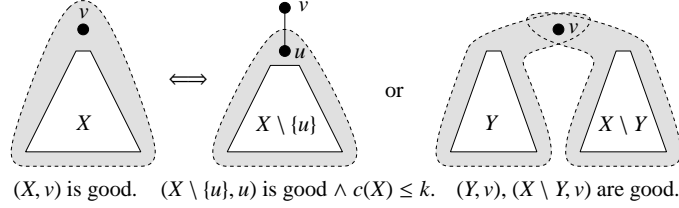
Fig. 3. An illustration of Lemma 4.2.
